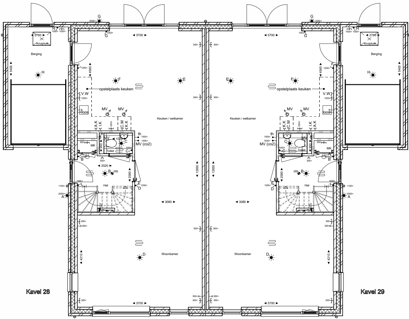
begane grond
