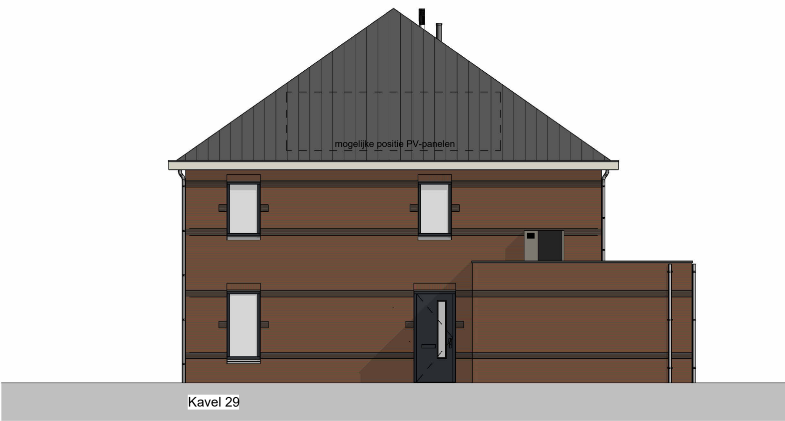
rechtergevel
