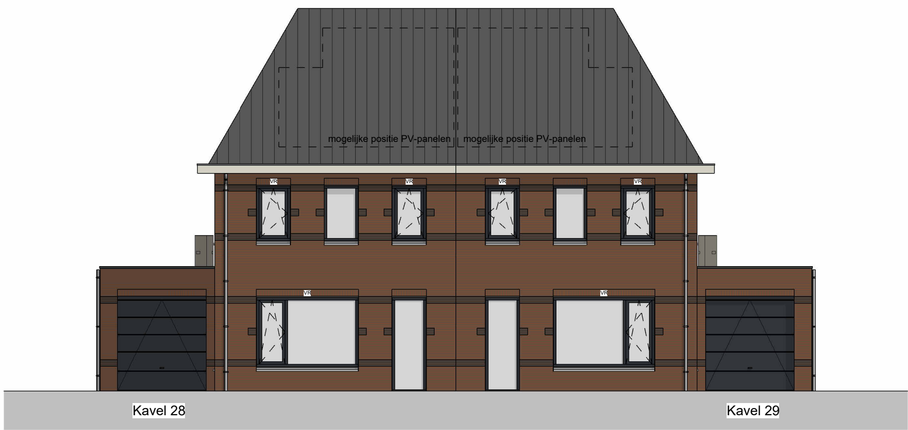
voorgevel
